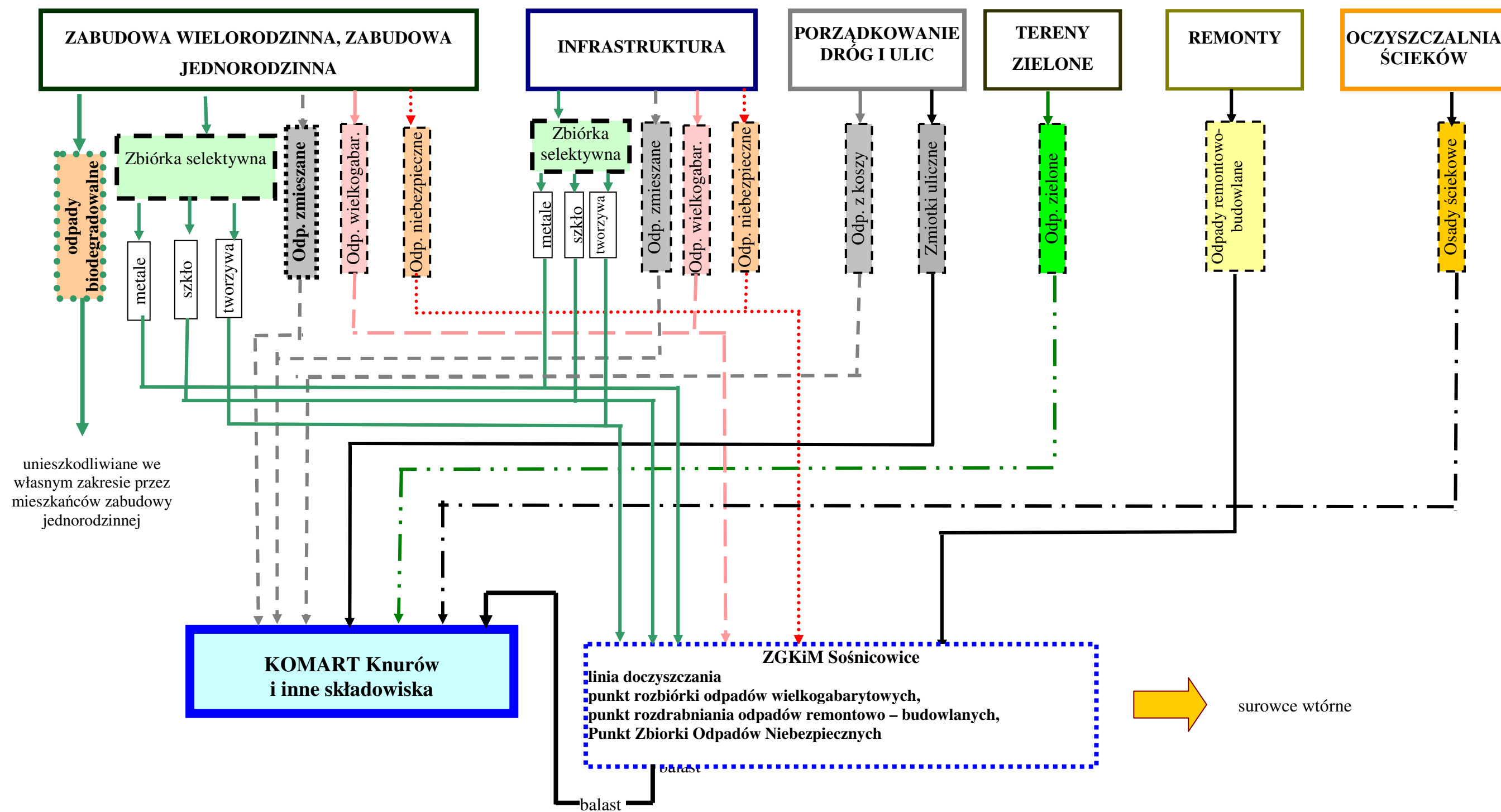
Rysunek 4. Schemat gospodarki odpadami na terenie gminy Sośnicowice po 2009 r. – Wariant I
